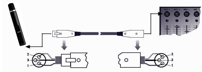
Figura 3: Conexión con cable XLR balanceado
